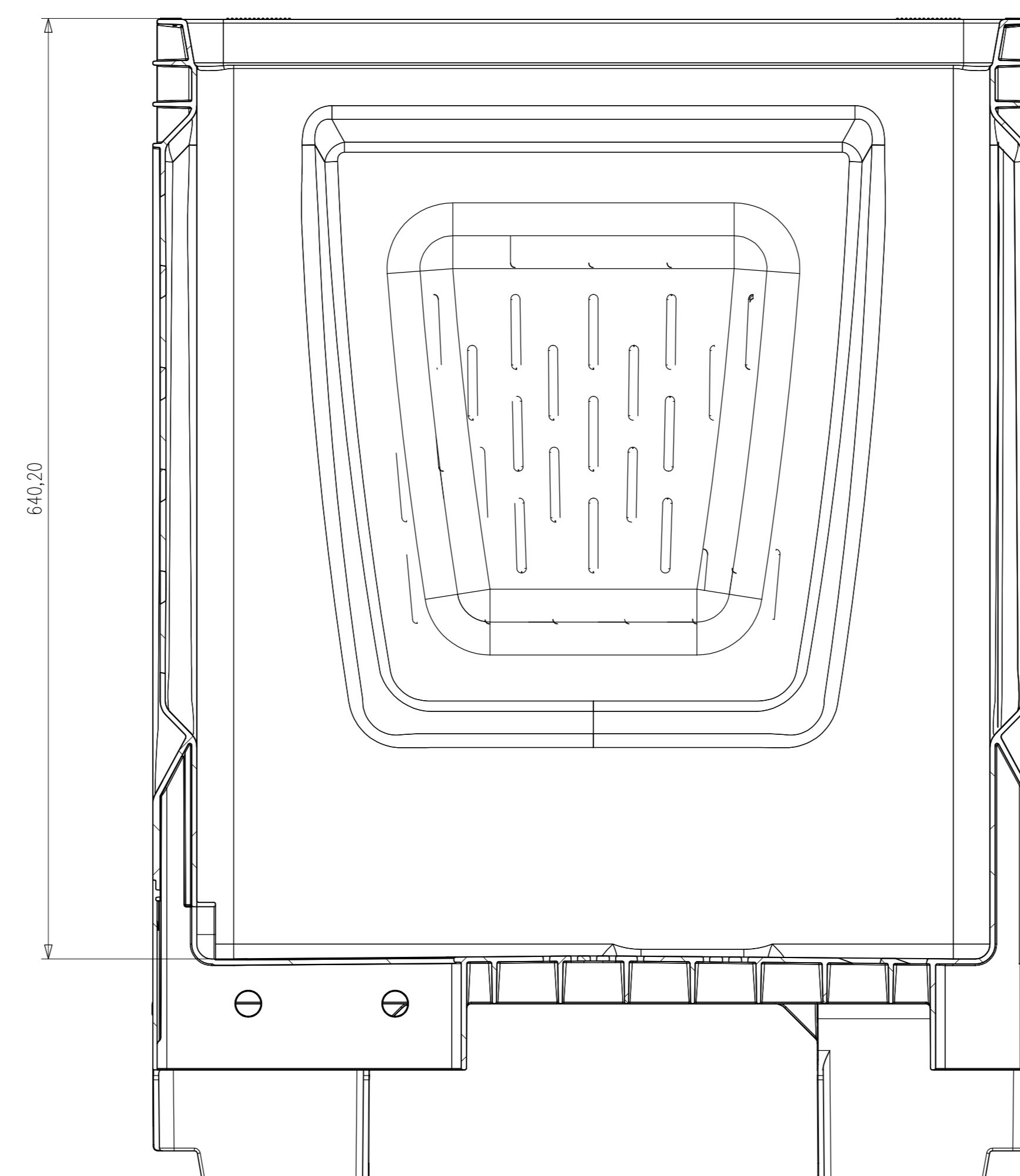
Schnitt A-A
