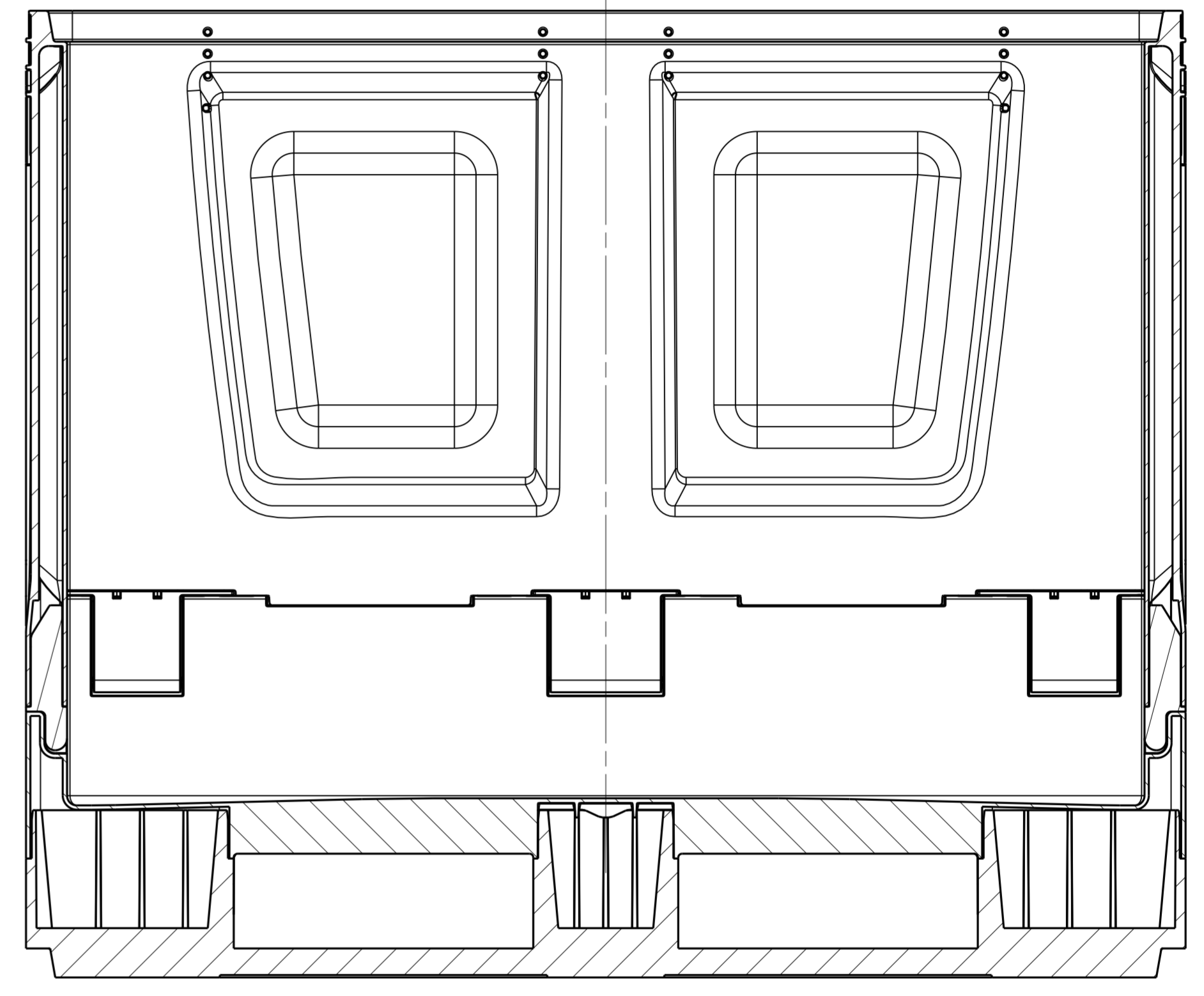
Schnitt B-B
